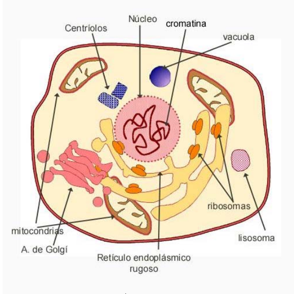
Célula Animal.
