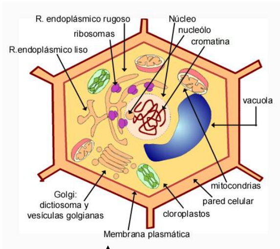
Célula Vegetal
